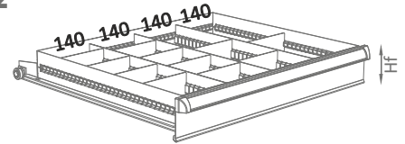
Ref. 122 Hf D2 Hf 075-100-125-150-200-250
