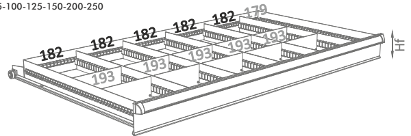
Ref. 143 Hf D6 Hf 075-100-125-150-200-250
