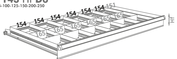
Ref. 143 Hf D6 Hf 075-100-125-150-200-250
