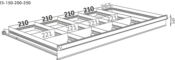
Ref. 143 Hf D5 Hf 075-100-125-150-200-250
