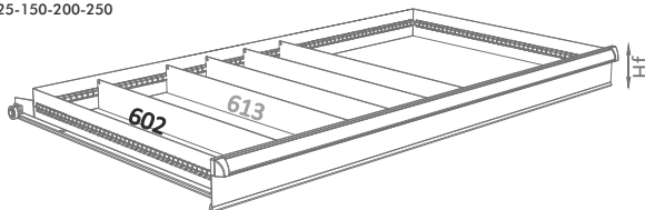
Ref. 143 Hf D5 Hf 075-100-125-150-200-250
