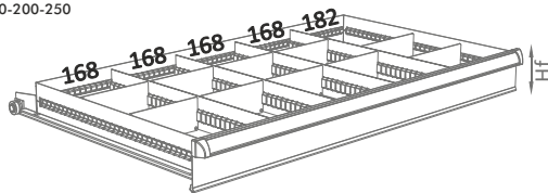
Ref. 123 Hf D2 Hf 075-100-125-150-200-250
